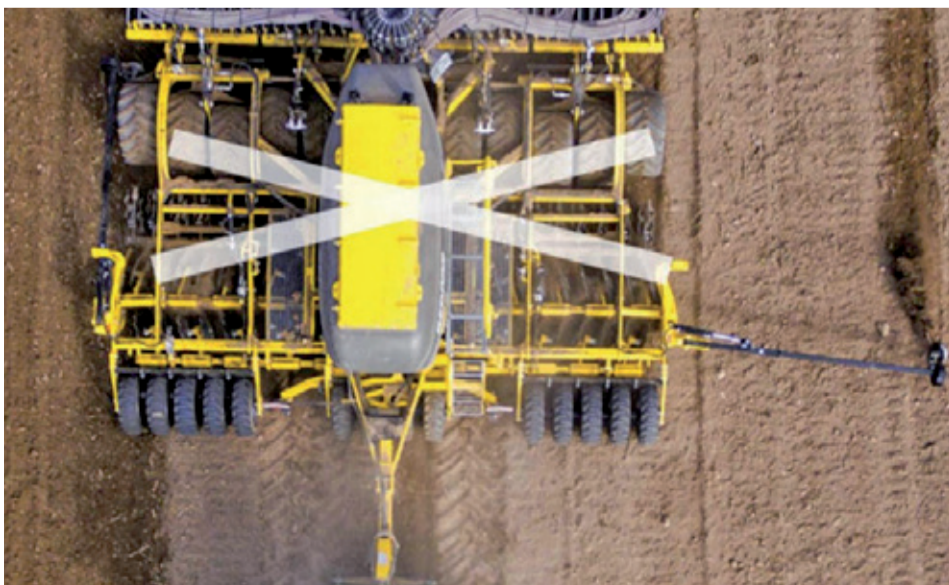
Disková sekcia sejacieho stroja OMEGA OO_L je navrhnutá s cieľom zamedziť bočnému posunu.
